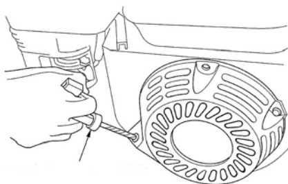
Abb. 21: Zugstarter betätigen
