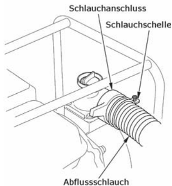
Abb. 15: Abflussschlauch anschließen
