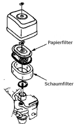
Abb. 11: Filter überprüfen
