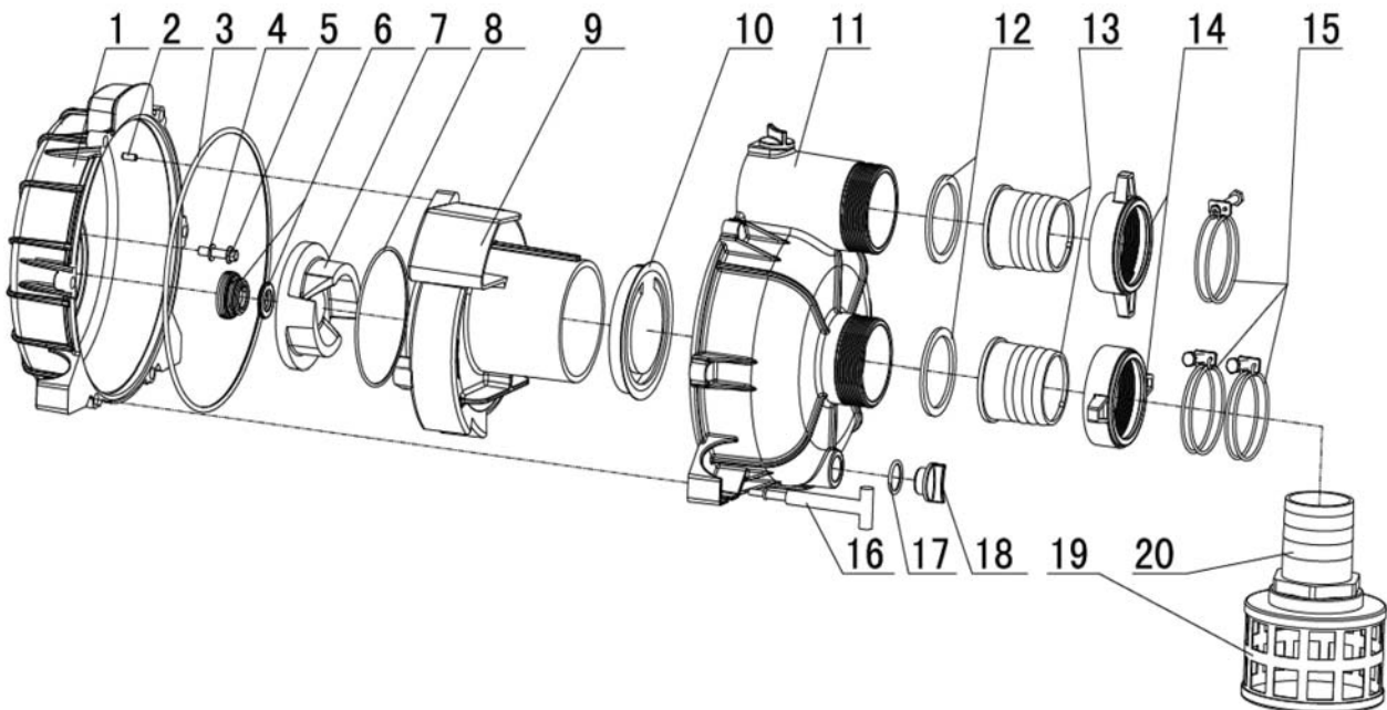
Abb. 30: Ersatzteilzeichnung 3 SWP 80
