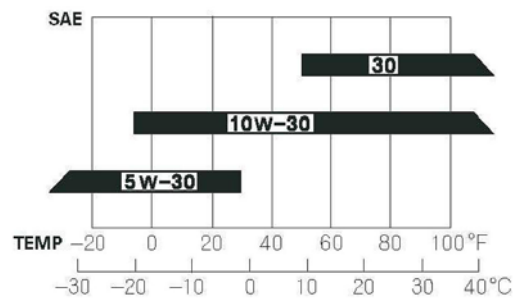
Abb. 24: Motoröl in Abhängigkeit der Temperatur
