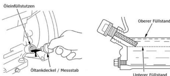
Abb. 10: Ölstand überprüfen
