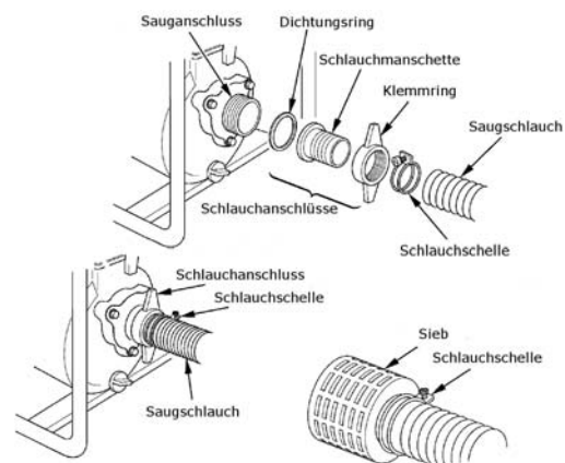
Abb. 14: Ansaugschlauch montieren
