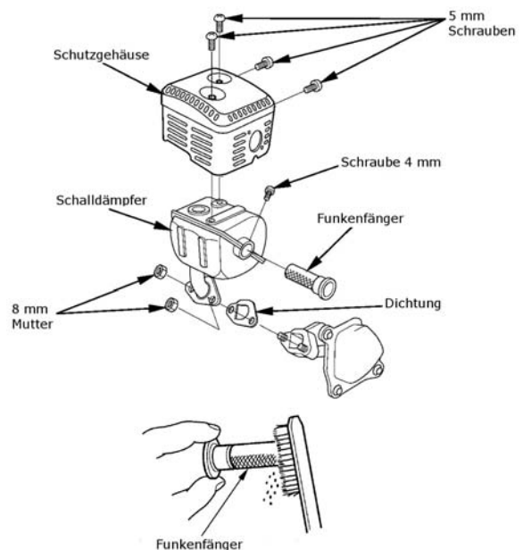
Abb. 26: Ausbauen Funkenfänger
