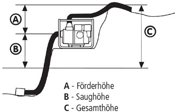
Abb. 13: Platzierung der Pumpe
