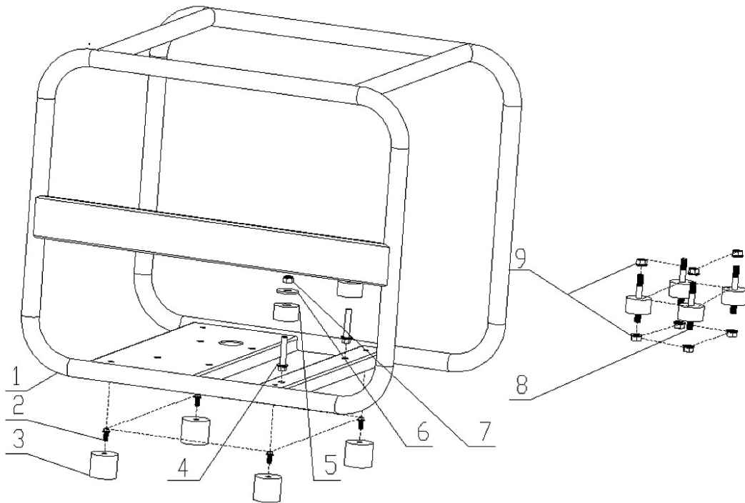
Abb. 29: Ersatzteilzeichnung 2 SWP 80
